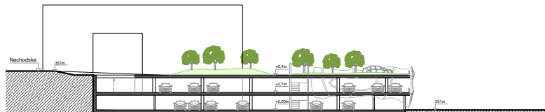
ŘEZ A-A'
