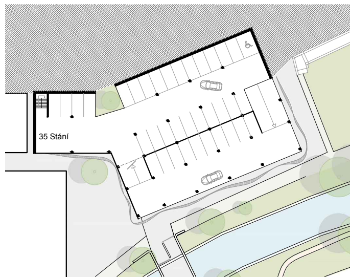
PARKING B 2,3 NP + 2,70 m
