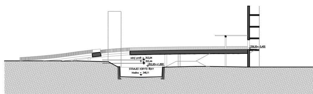
ŘEZ C-C'
